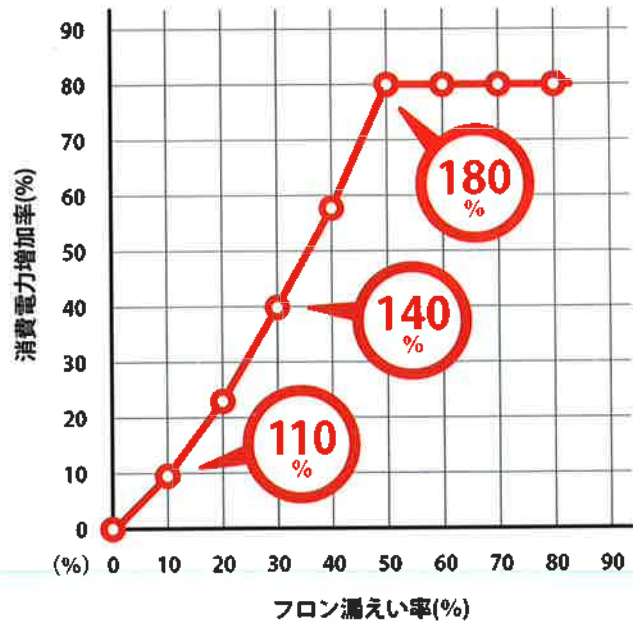
統一的な評価で用いるフロン漏えい率と消費電力増加率の関係
